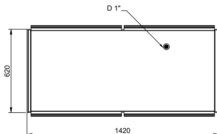
Boven aanzicht
